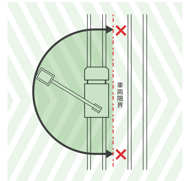
(例) 選択スイッチを左に入れることで 車両左側のみブーム旋回が可能
