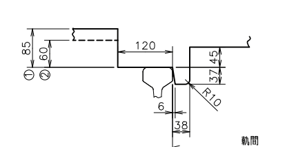
車輪に対する車両限界寸法
